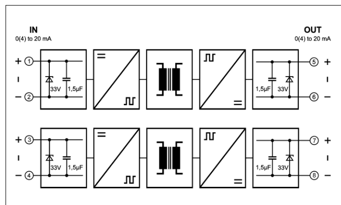
Prinzipschaltbild
